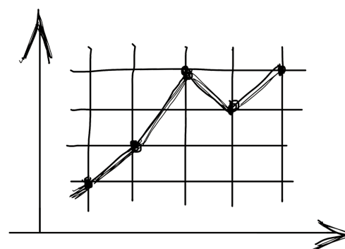
Стоимость функций
