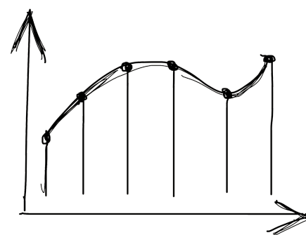
Стоимость пакетов
